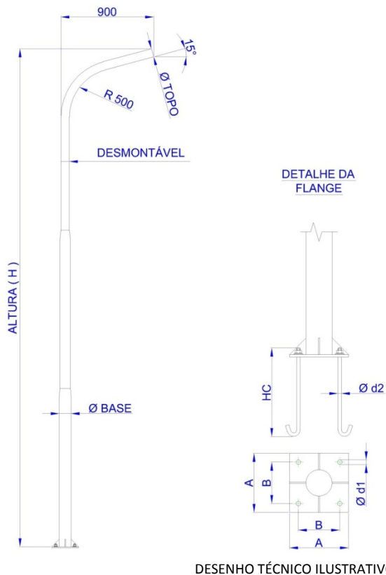
DESENHO TÉCNICO ILUSTRATIVO
