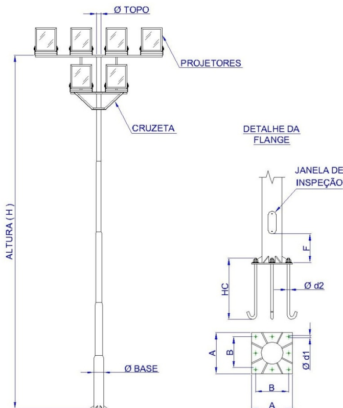
DESENHO TÉCNICO ILUSTRATIVO
